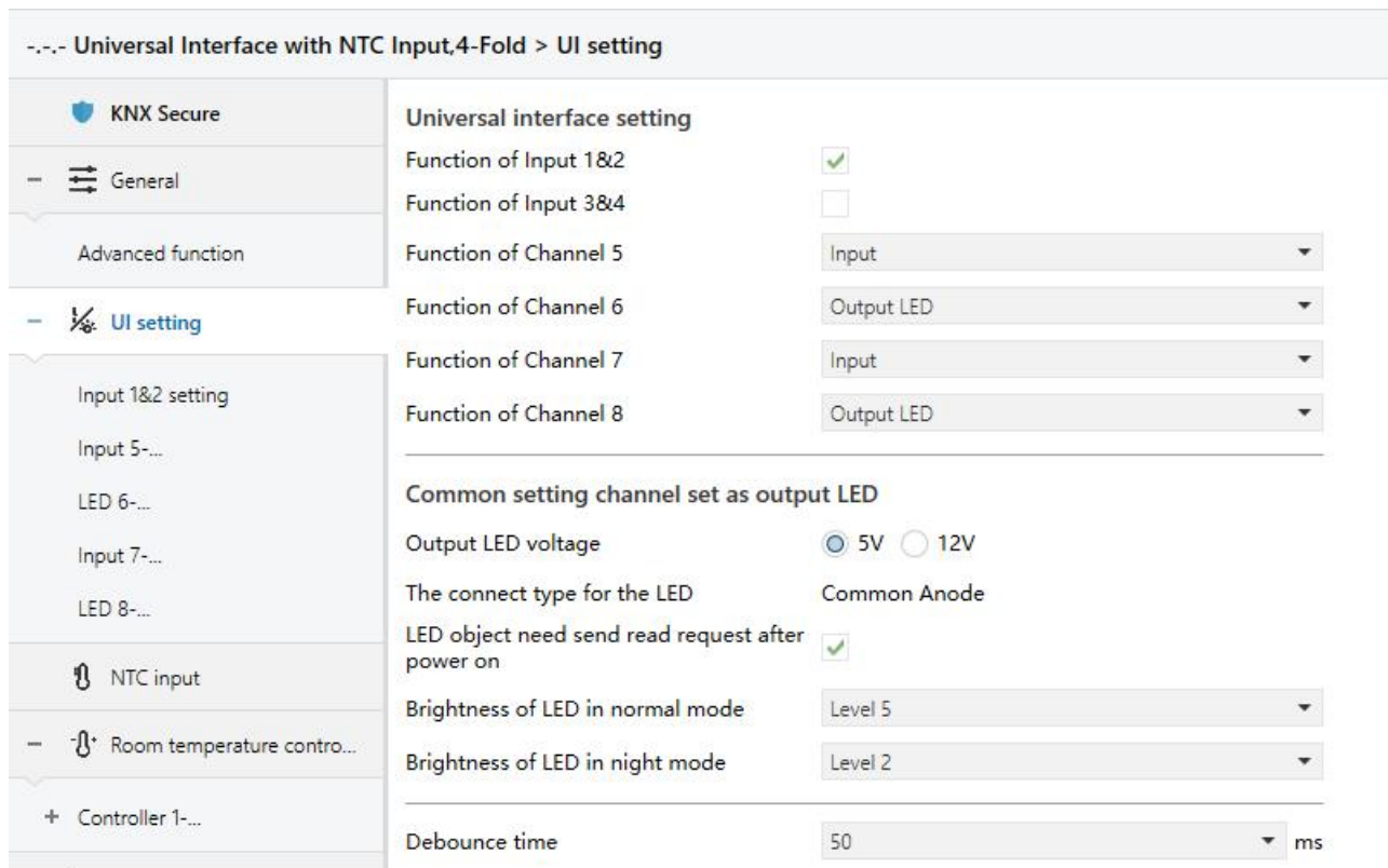
图 4.6 参数设置界面 “UI setting”
