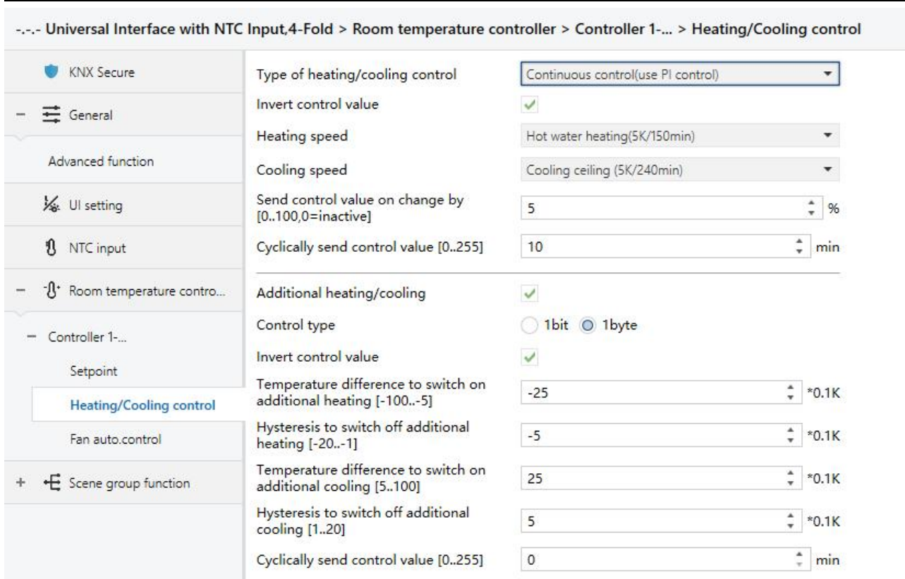
图 4.3.1.2 参数设置界面 “Heating control/Cooling control/Heating/Cooling control”
