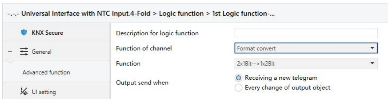
图 4.4.4 “Logic function _Format convert” 功能参数
