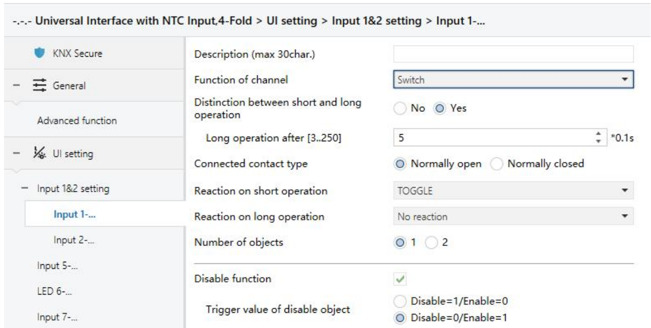
图 4.6.2.1 功能参数 “Input x-Switch”
