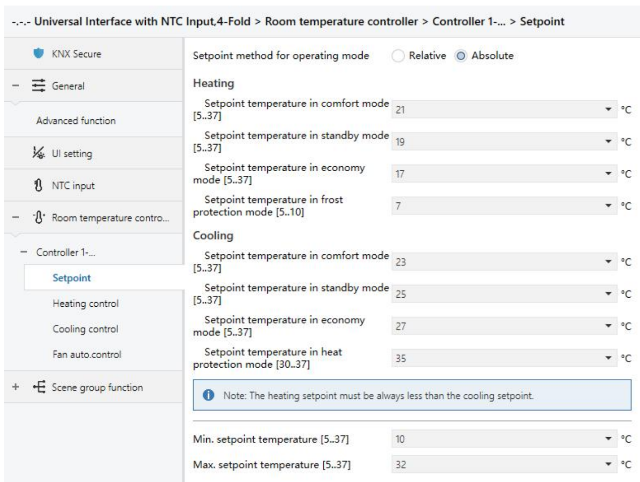
图 4.3.1.1 参数设置界面 "Setpoint"
