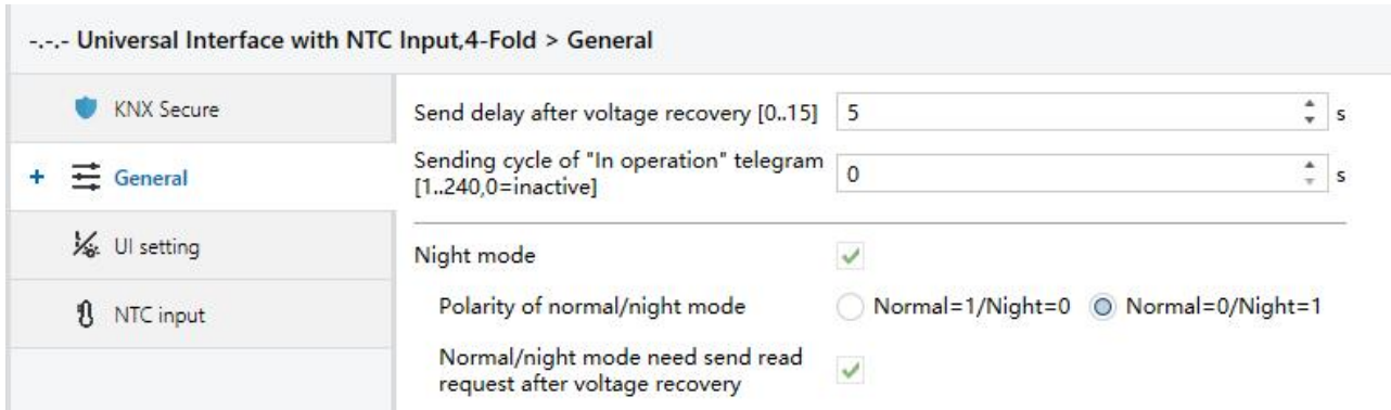
图 4.2 参数设置界面 “General”
