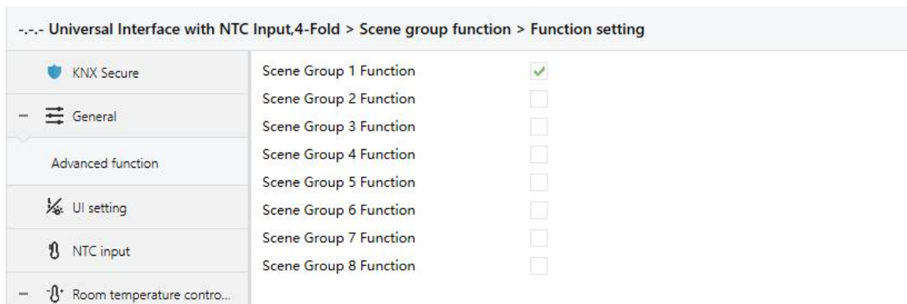
4.5(1)参数设置界面 “Scene Group function”
