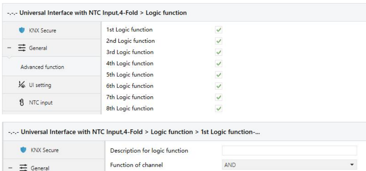
图 4.4 参数设置界面 “Logic function”
