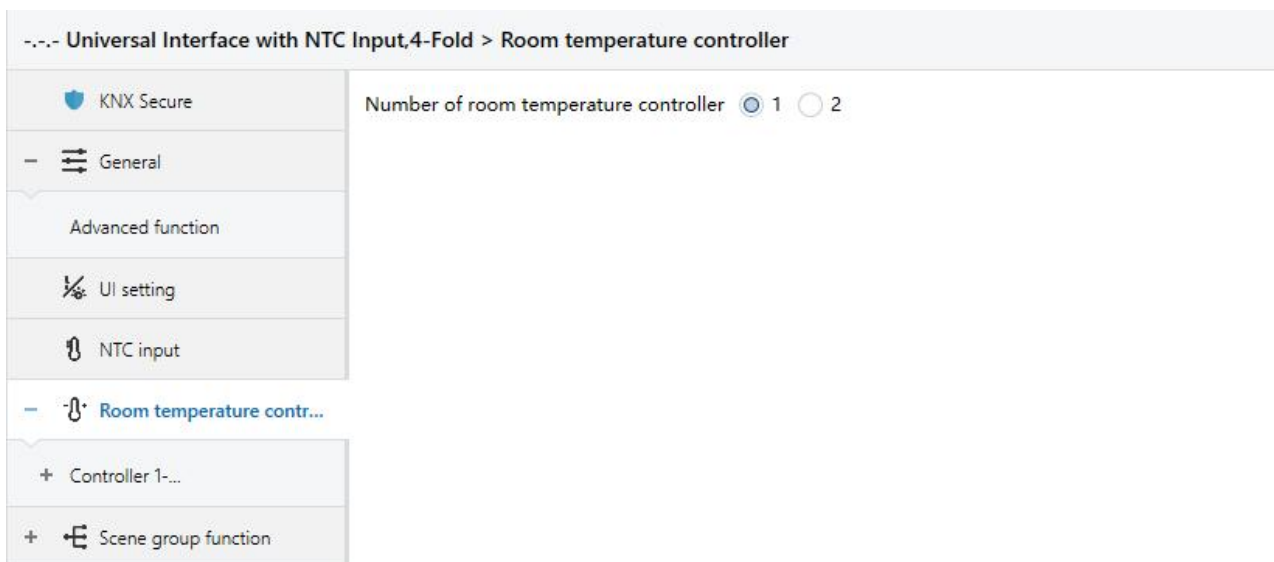
图 4.3 参数设置界面 “Room temperature controller”
