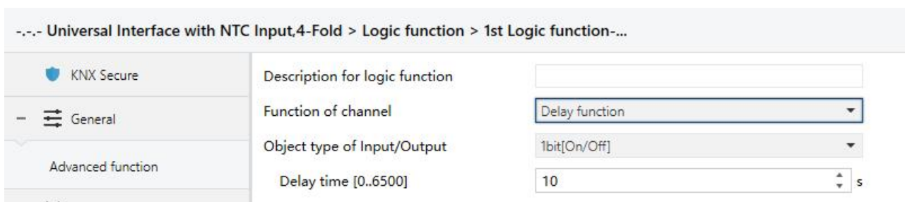
图 4.4.6 “Logic function _Delay function” 功能参数
