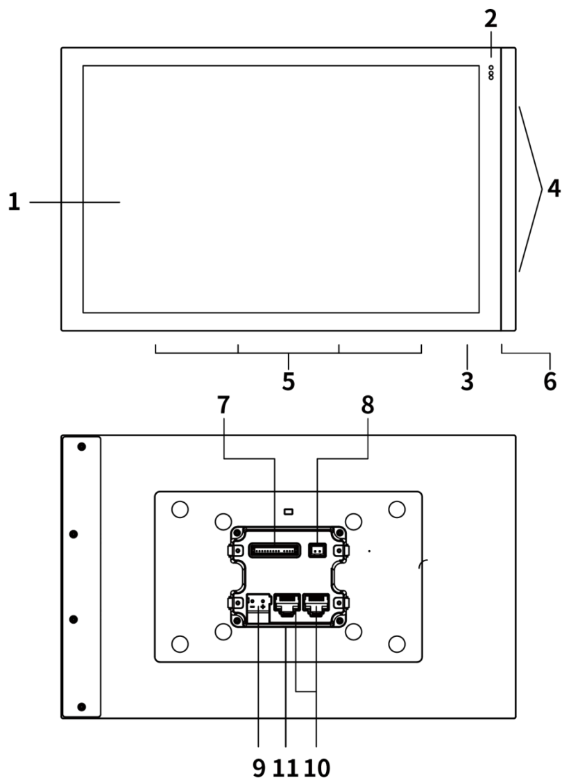
图 3.2.1 KNX 智能屏 S13
