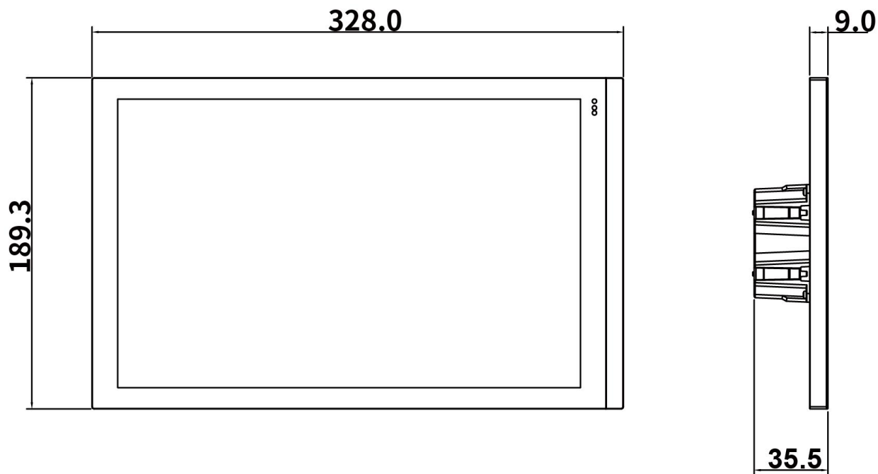
图 3.1.1(1) KNX 智能屏 S13
