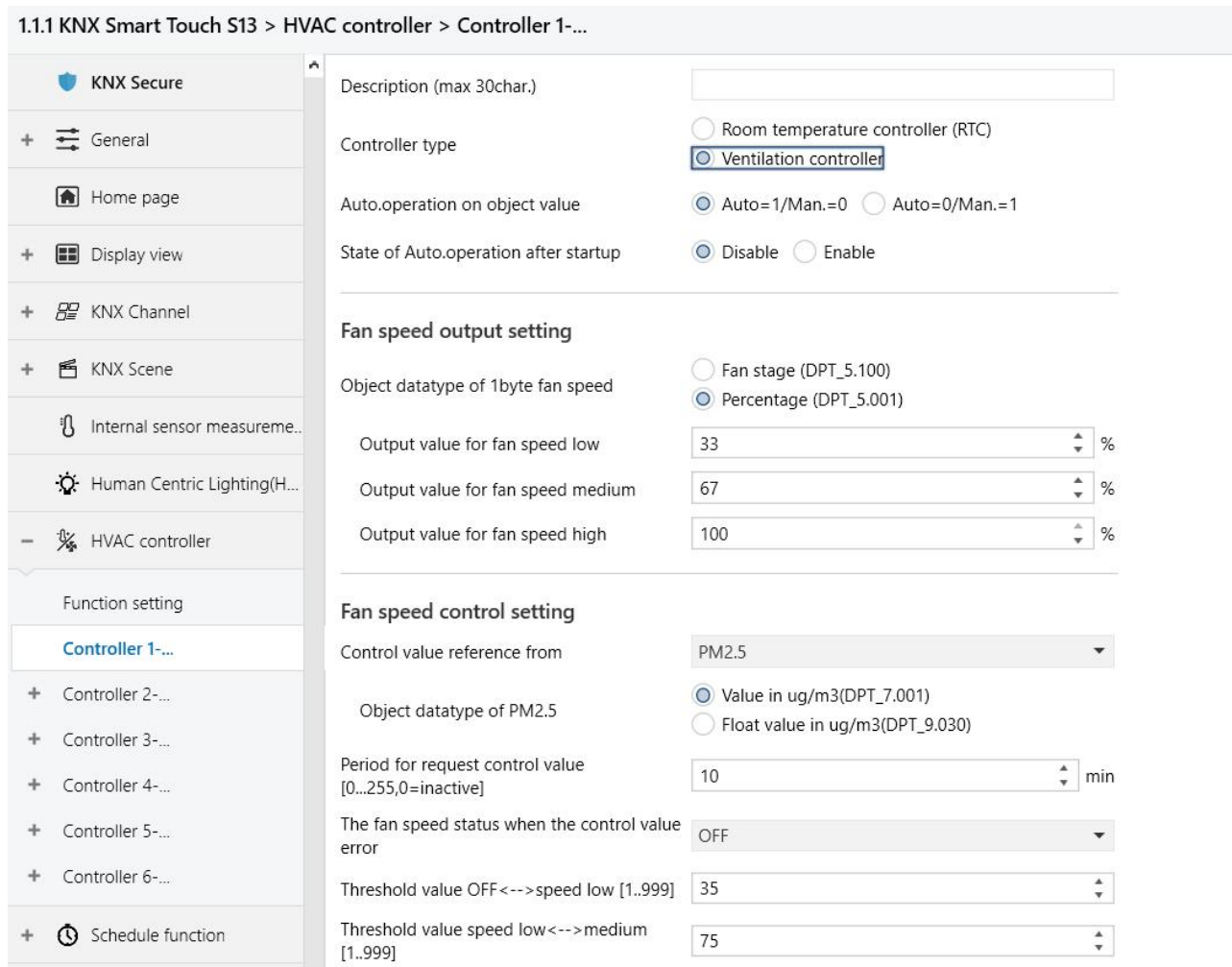
Fig.5.3.2 "Cotroller x-Ventilation controller"(x=1~6) parameter window
