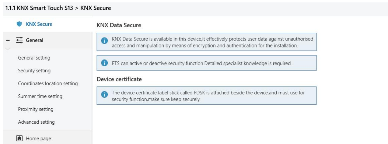
Fig.5.1 (1) "KNX Secure" parameter window
