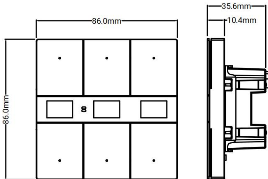
面板尺寸图
