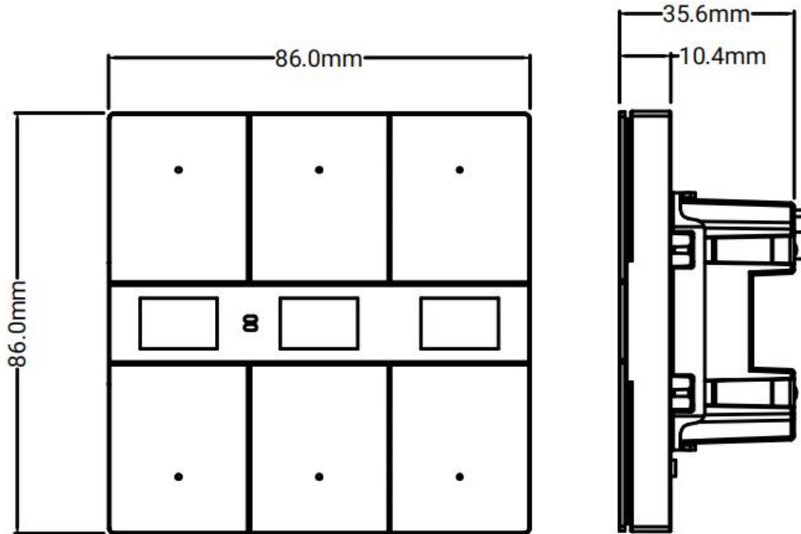
面板尺寸图
