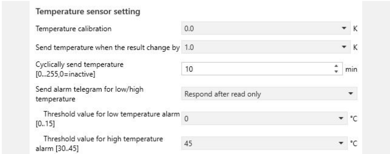
图 5.3 “Internal temperature measurement” 参数设置界面
