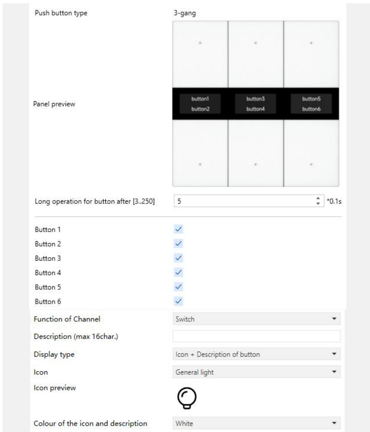
图 5.4 “Button” 参数设置界面
