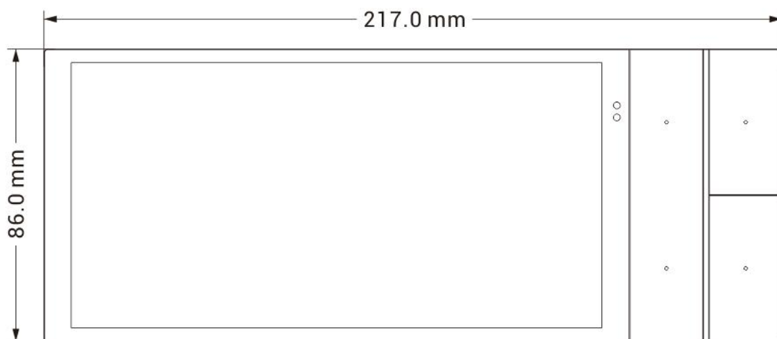
图 3.1.1(2) KNX 智能屏 S7 带四键子面板-底座
