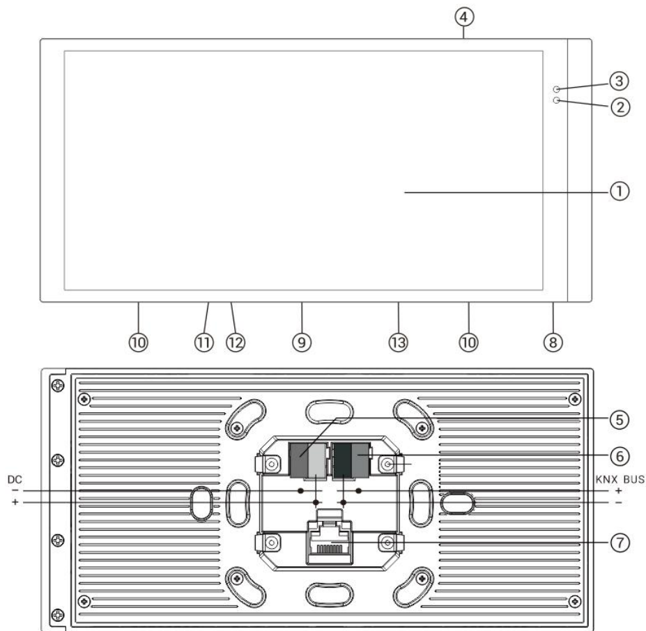
图 3.2.1 KNX 智能屏 S7
