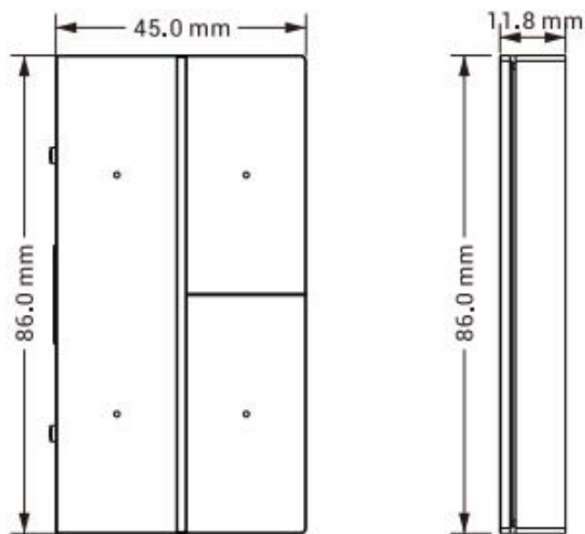
图 3.1.2 S7 四键子面板-底座
