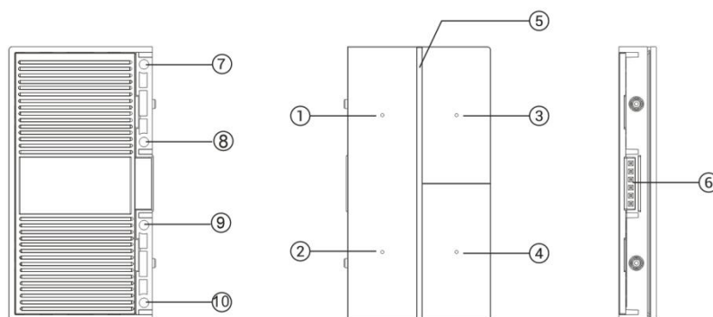
图 3.2.2 S7 四键子面板-底座
