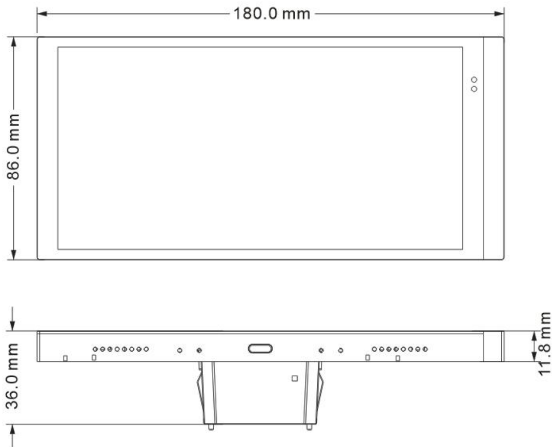
图 3.1.1(1) KNX 智能屏 S7
