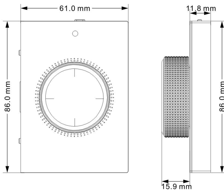
图 3.1.3 S7 旋钮子面板
