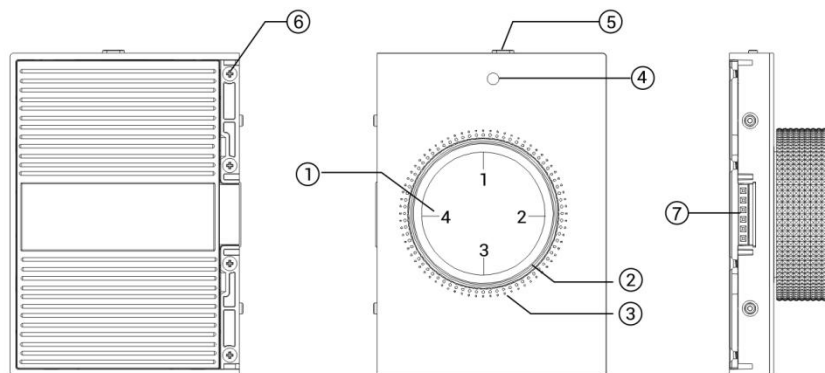
图 3.2.3 S7 旋钮子面板
