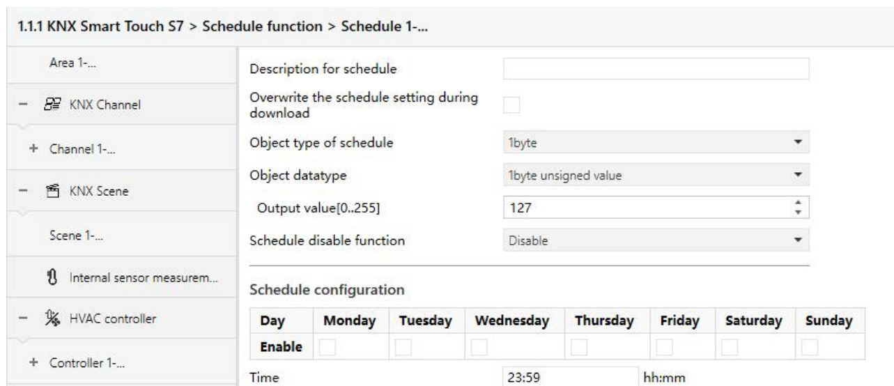
图 5.5.1 “Schedule X”参数设置界面
