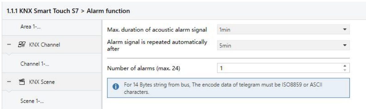
图 5.6 “Alarm function”参数设置界面
