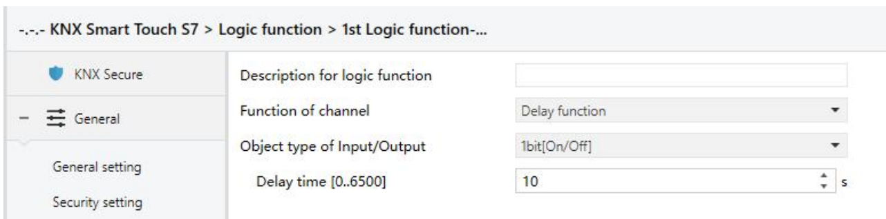
图 5.7.6 “Delay function”功能参数
