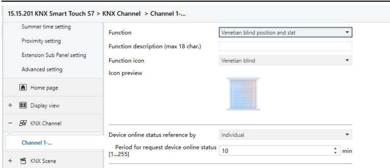
图 5.11.2(6)窗帘功能参数设置界面
