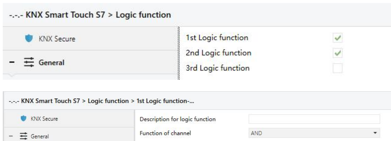
图 5.7 “Logic function”参数设置界面
