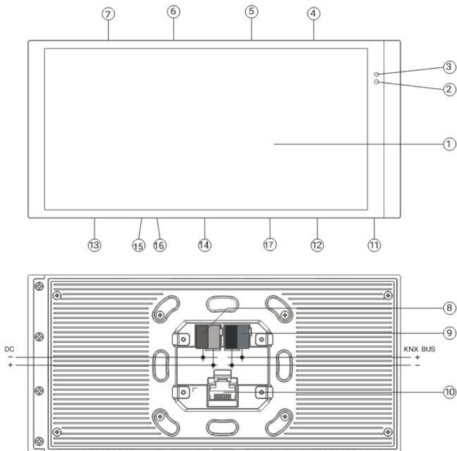
图 3.2.1 KNX 智能屏 S7
