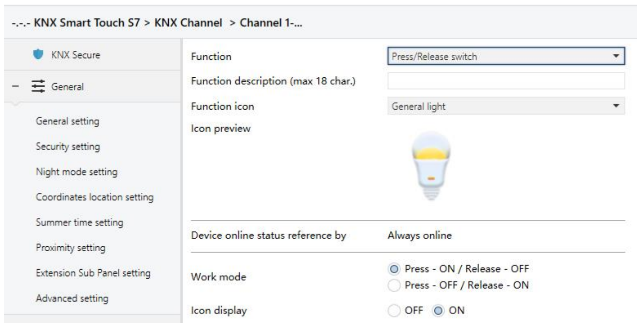
图 5.11.2(2) 按下/松开开关功能参数设置界面
