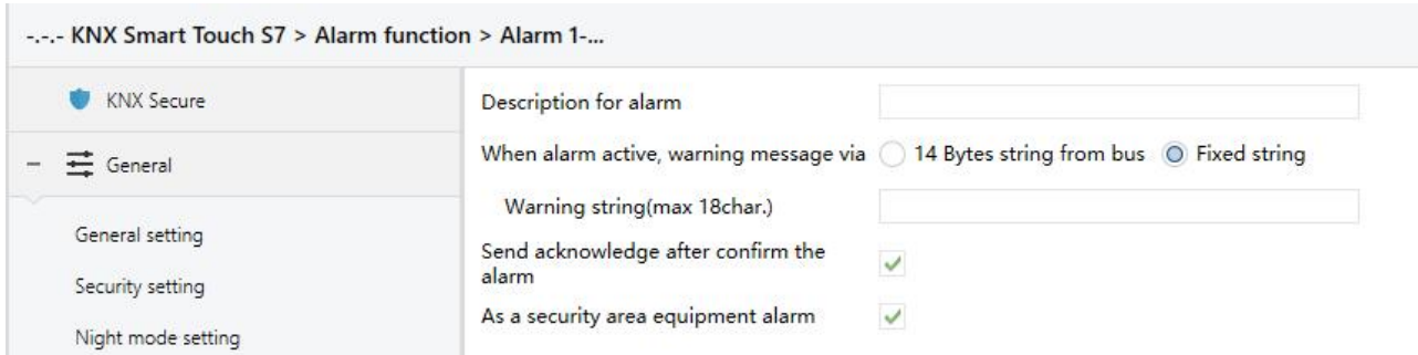
图 5.6.1 “Alarm x”(x=1~24) 参数设置界面
