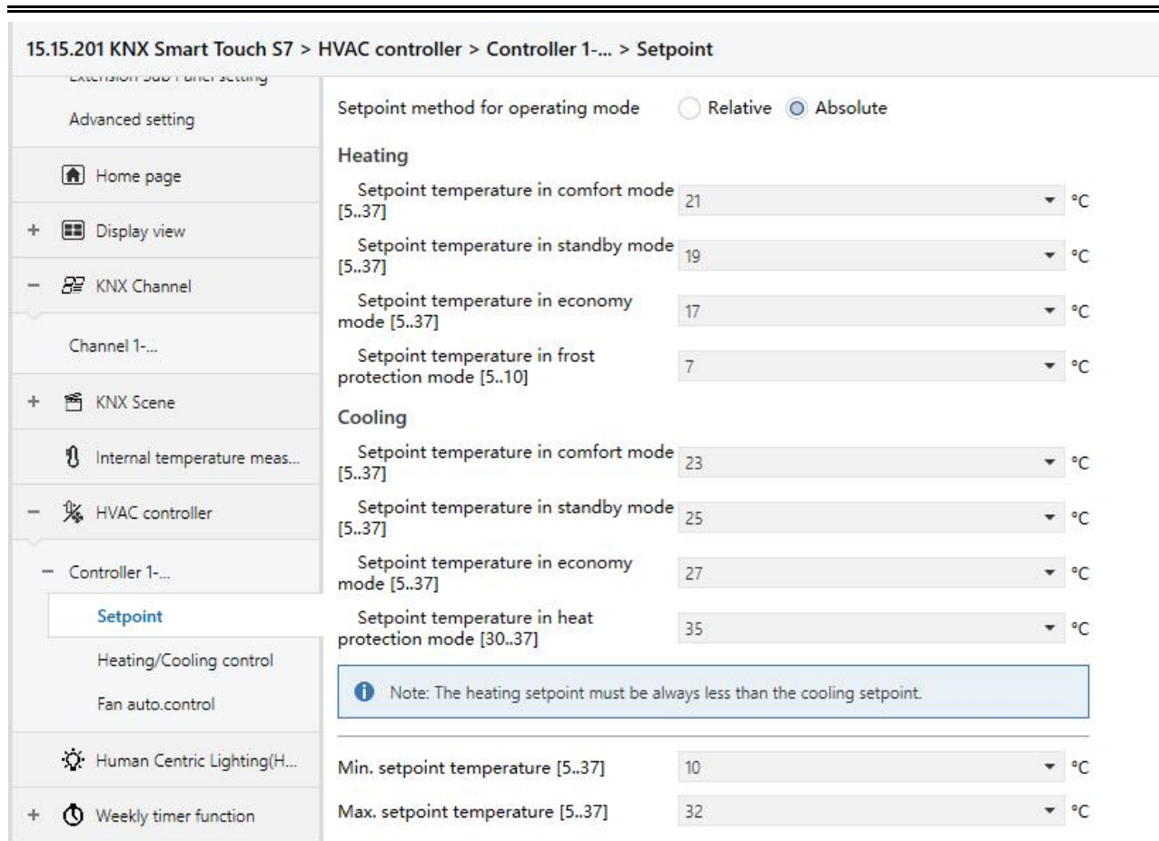
图 5.3.1.1“Setpoint”参数设置界面
