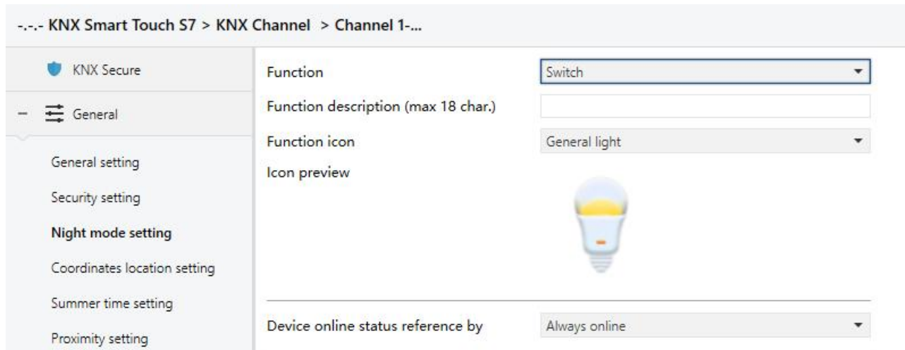
5.11.2(1) 开关功能参数设置界面
