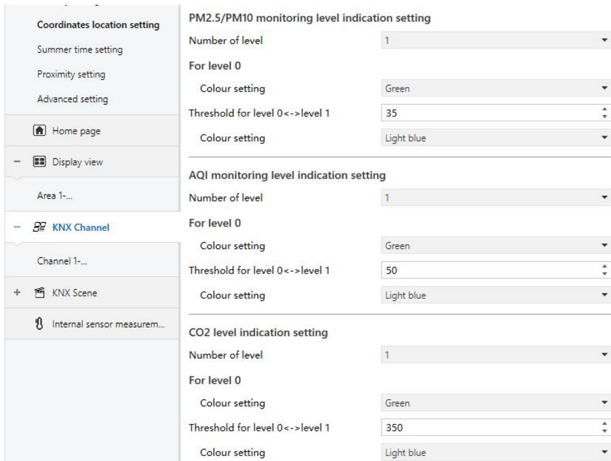
图 5.11 “KNX Channel”参数设置界面
