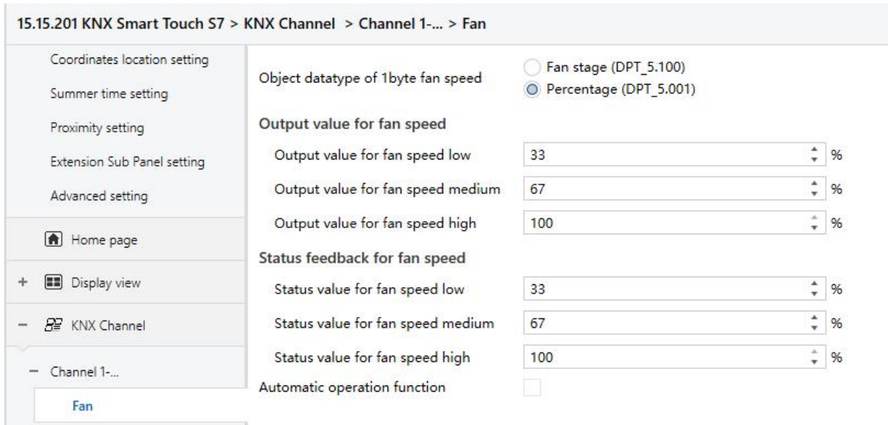
图 5.11.2.1(9) Fan 参数设置
