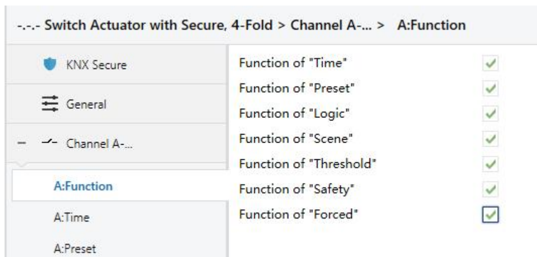
Fig. 4.4(2) Starting parameter window "X: Function"
