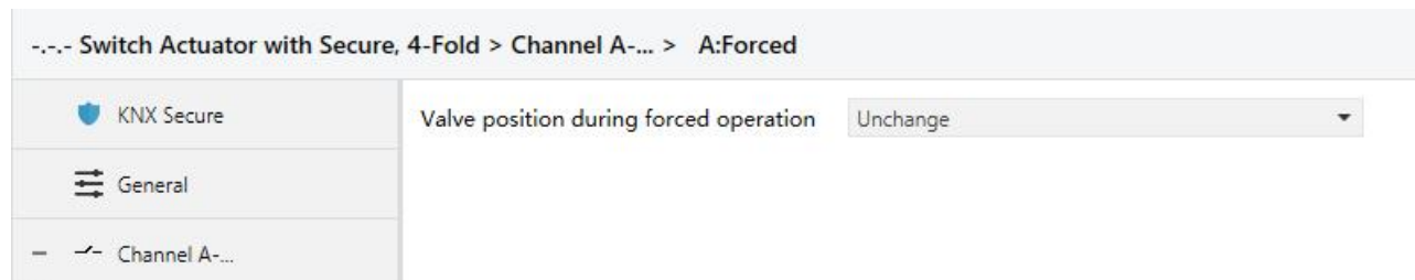
Fig. 4.5.2 Parameter window "X: Forced"
