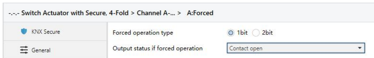
Fig. 4.4.7 Parameter window "X: Forced"
