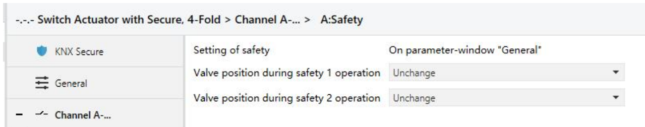
Fig. 4.5.4 Parameter window "X: Safety"
