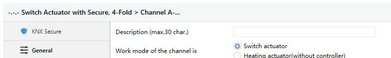
Fig.4.3 Parameter window "Channel X"
