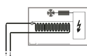
2-pipe fan coil
