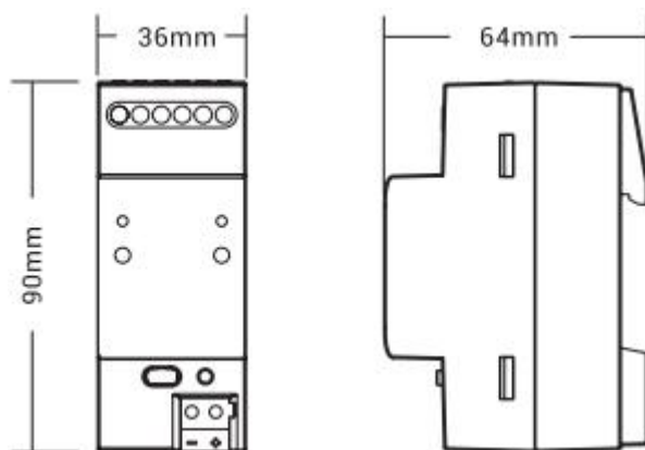
1 路尺寸图
