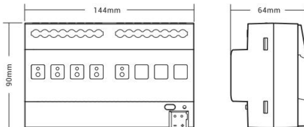
4 路尺寸图
