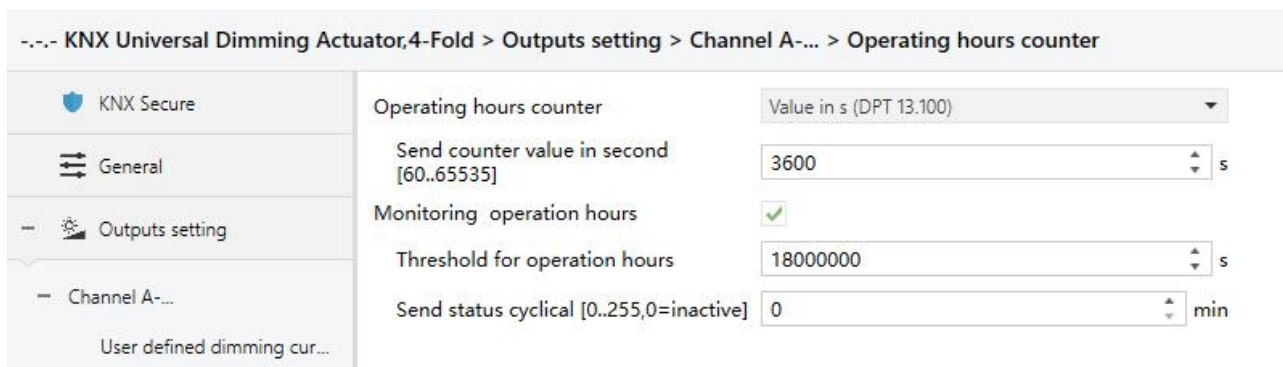
图 5.3.3.6 “Operating hours counter” 参数设置界面
