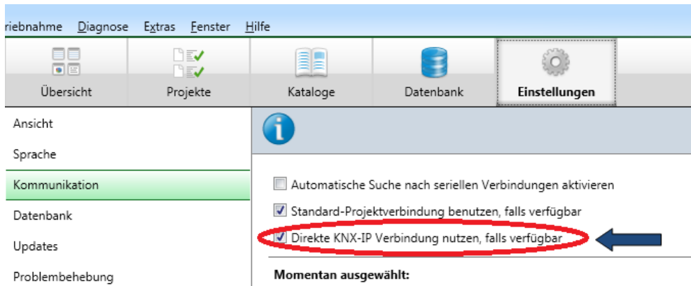
Abbildung 10: Die Einstellung „ Direkte KNX-IP-Verbindung nutzen, falls verfügbar “ beschleunigt die Übertragung von der ETS zum Gerät.
