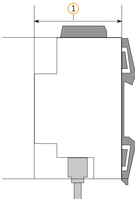
Abbildung 14: Gerät seitlich
