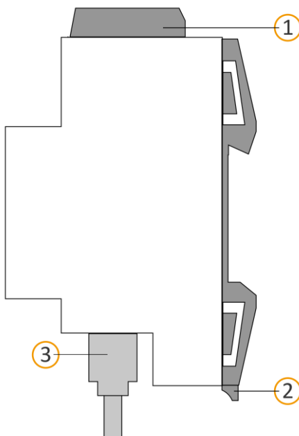
Abbildung 11: Gerät seitlich inklusive Abdeckkappe und verbundenem RJ45-Kabel
