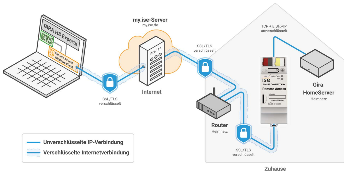
Abbildung 27: Sichere Konfiguration des Gira HomeServers per Fernwartung
