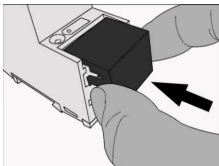
Abbildung 14: Abdeckkappe aufstecken
