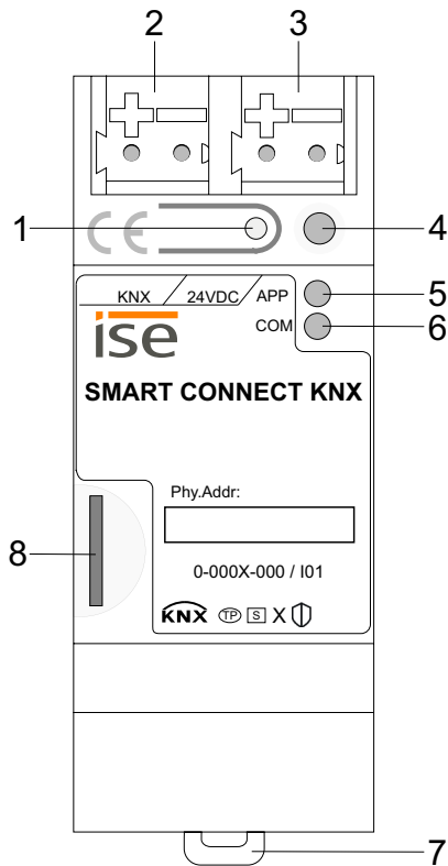
Abbildung 4: Vorderseite
