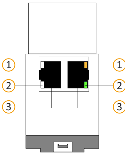
Abbildung 7: Netzwerkanschlüsse
