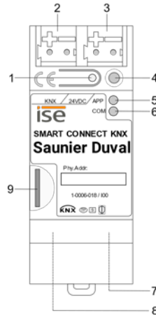
Abbildung 9: ise smart connect KNX Saunier Duval.
