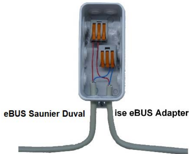
Abbildung 4: Abzweigdose zur Anbindung des ise eBUS Adapters an das Heizungssystem.
