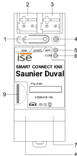
Abbildung 1: ise smart connect KNX Saunier Duval
