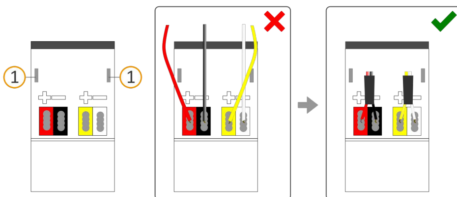
Abbildung 11: Kabelführung
