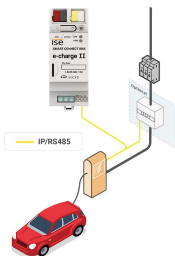
Abbildung 26: Stromzähler am Ladepunkt
