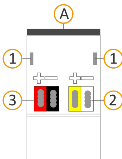
Abbildung 5: Geräteoberseite
