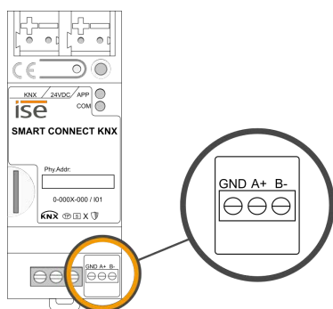
Abbildung 14: Belegung Schraubklemme
