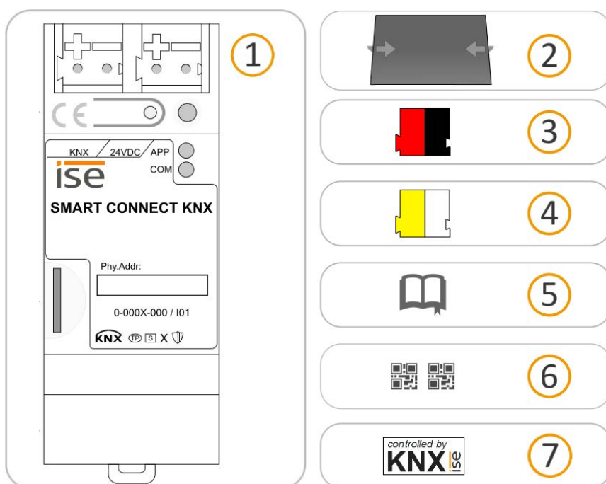
Abbildung 8: Lieferumfang
