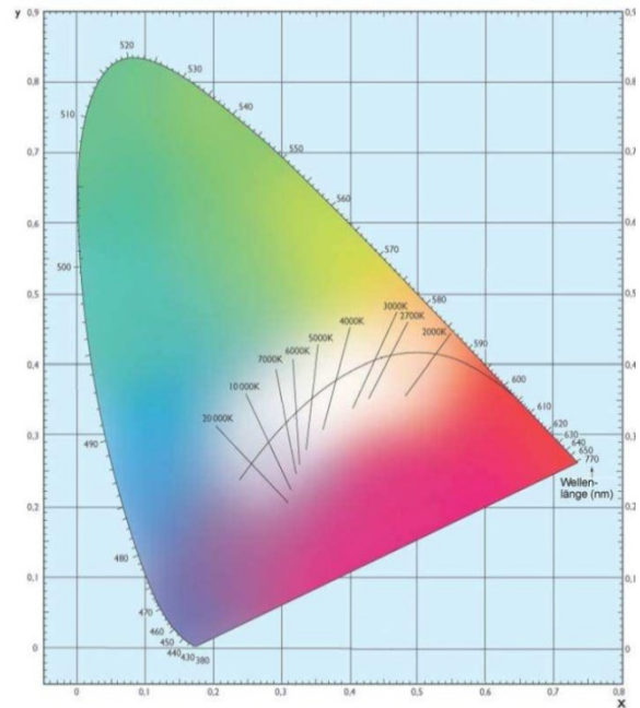
Abbildung 1: Farbraum-Chromatizitäts-Diagramm nach CIE 1931 (Quelle: Wikipedia)
