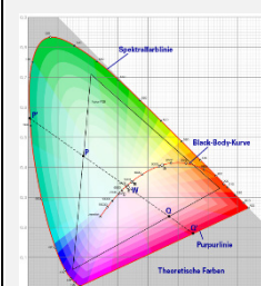
Abbildung 8: XY-Farbraum (Quelle: Wikipedia)
