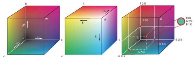
Abbildung 4: RGB Würfel (Quelle: Wikipedia)
