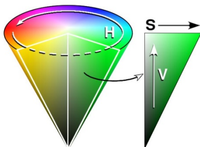
Abbildung 5: HSV-Farbraum (Quelle: Wikipedia)
