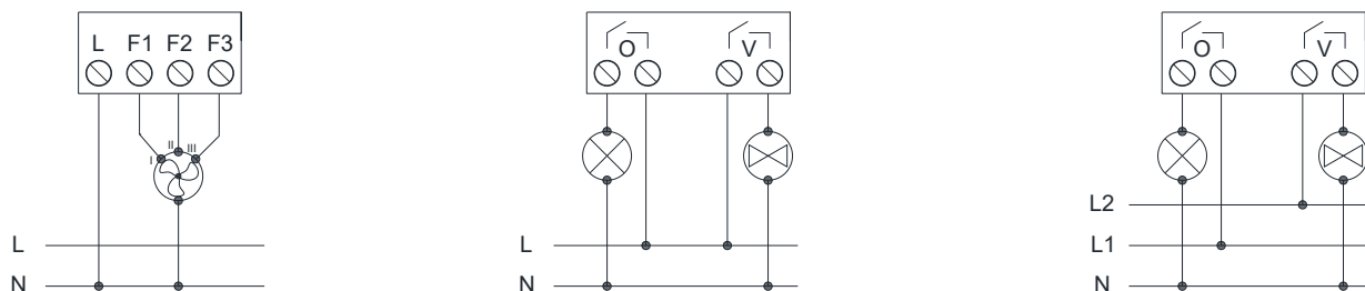
Figura 2: Ejemplo de conexionado (de izquierda a derecha): ventilador con 3 velocidades, carga y válvula todo-nada, carga y válvula todo-nada a fases distintas.
