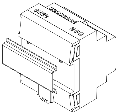
Figura 3: Montaje de ALLinBOX Hospitality v2 en carril DIN
