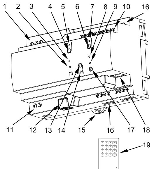
Figura 1: ALLinBOX 88 v2
