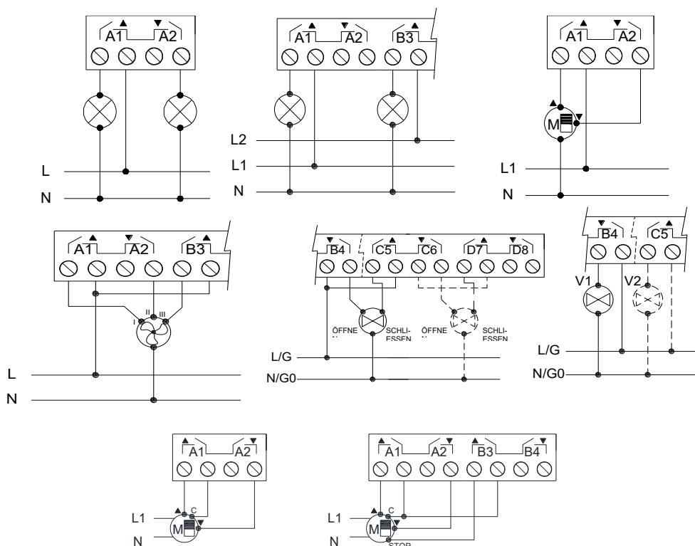
Abbildung 2: Anschlussbeispiel (von links nach rechts und von oben nach unten): 2 Lasten, 2 Lasten in verschiedenen Phasen, Jalousie, Fan Coil mit 3 Geschwindigkeiten, Dreipunkt-Fan-Coil-Ventile, Alles-oder-Nichts- Fan-Coil-Ventile, eine Jalousie mit zwei potentialfreien Kontakten und eine Jalousie mit drei potentialfreien Kontakten
