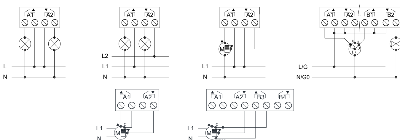
Figure 2 : Exemples de connexions (de gauche à droite et de haut en bas) : 2 charges, 2 charges avec différentes phases, volets, ventilateur avec 3 vitesses, vannes de ventilo-convecteur tout-ou-rien, un volet de 2 contacts secs et un volet de 3 contacts secs.
