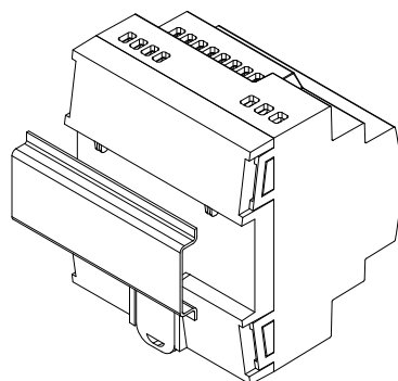
Figura 3: Montaje de ALLinBOX 46 v2 en carril DIN
