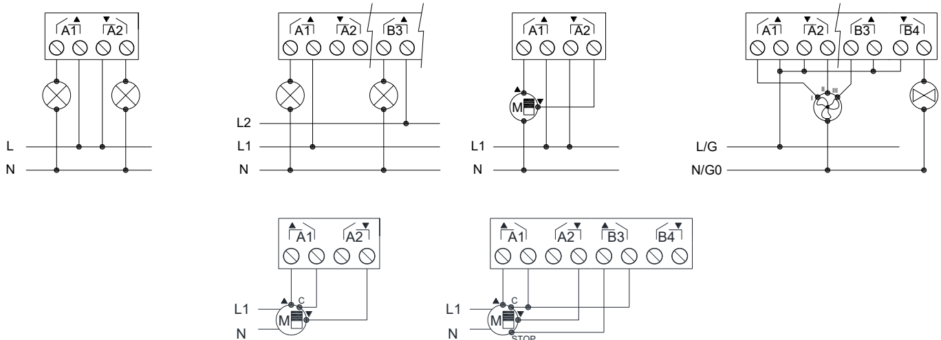
Abbildung 2: Anschlussbeispiel (von links nach rechts und von oben nach unten): 2 Lasten, 2 Lasten in verschiedenen Phasen, Jalousie, Ventilator mit 3 Geschwindigkeiten, Alles-oder-Nichts-Fan-Coil-Ventile, eine Jalousie mit zwei potentialfreien Kontakten und eine Jalousie mit drei potentialfreien Kontakten
