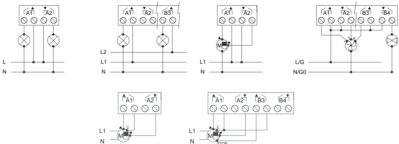
Figura 2: Ejemplo de conexionado (de izquierda a derecha, y de arriba a abajo): 2 cargas, 2 cargas a fases distintas, persiana, ventilador con 3 velocidades, válvulas todo-nada para fan coil de dos tubos, una persiana de dos contactos secos y una persiana de tres contactos secos
