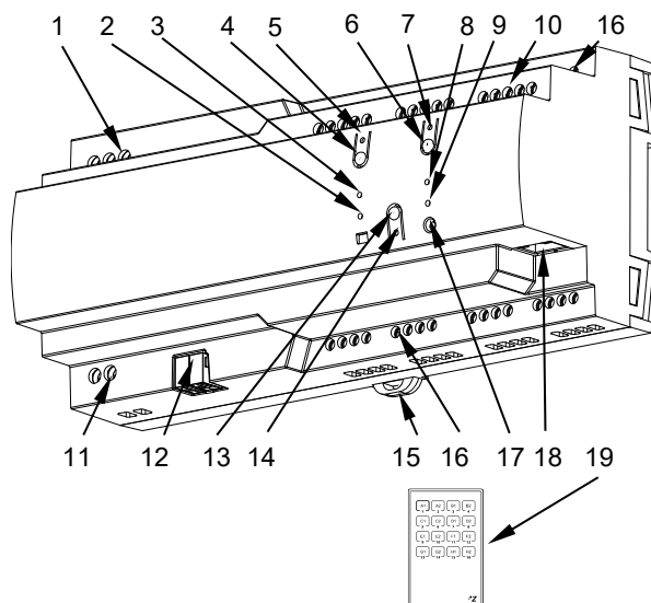
Figura 1: ALLinBOX 1612 v3
