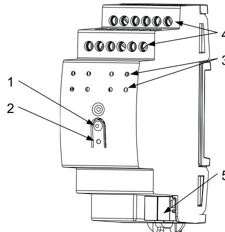
Abbildung 1: RailQUAD 8 v2
