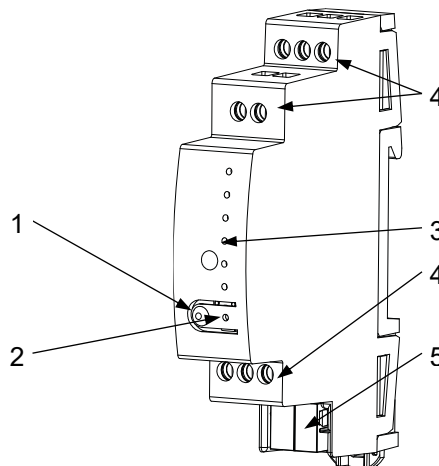
Abbildung 1: RailQUAD 6
