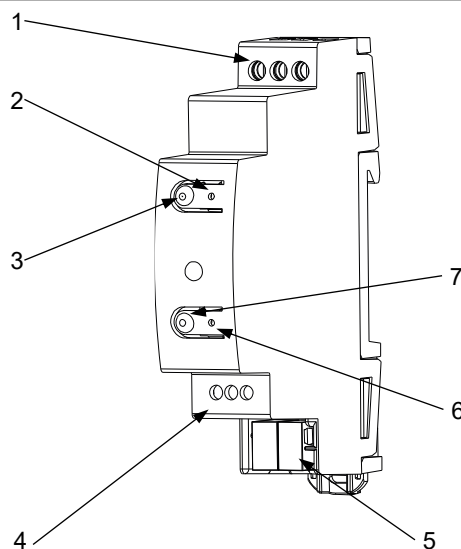
Figura 1: MicroBOX 12
