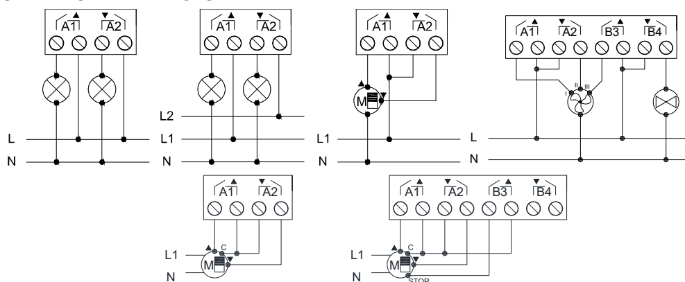
Figure 2 : Exemples de connexions (de gauche à droite et de haut en bas) : 2 charges, 2 charges sur différentes phases, volets, ventilo-convecteur, volets avec 2 contacts secs, volets avec 3 contacts secs.
