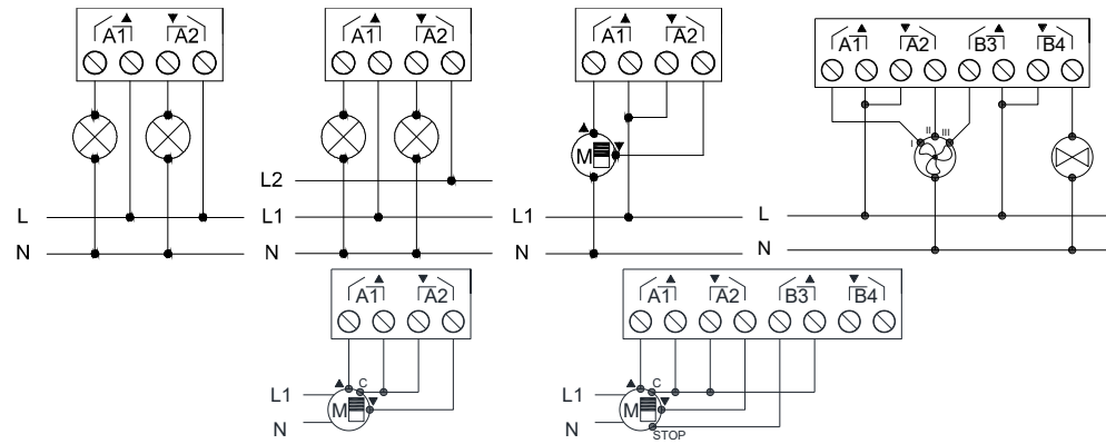
Figure 2 : Exemples de connexions (de gauche à droite et de haut en bas) : 2 charges, 2 charges sur différentes phases, volets, ventilateur-convecteur, volets avec 2 contacts secs, volets avec 3 contacts secs.
