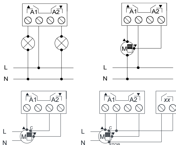
Figura 2. Ejemplo de conexionado (de izquierda a derecha): 2 cargas individuales, canal persiana, persiana con 2 contactos secos, persiana con 3 contactos secos.
