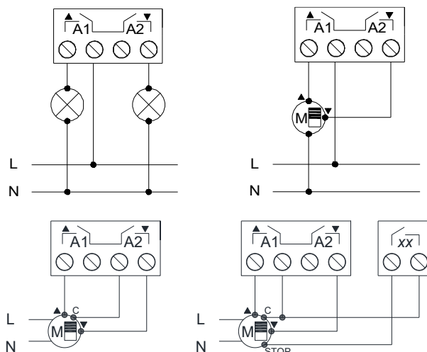
Abbildung 2. Anschlussbeispiel (von links nach rechts): 2 Einzelverbraucher, Rollladenkanal, Rollladen mit 2 potentialfreien Kontakten, Rollladen mit 3 potentialfreien Kontakten.
