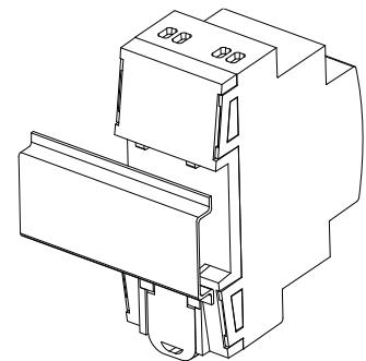
Abbildung 3: Montage der MINiBOX 0-10V X2 auf DIN-Schiene
