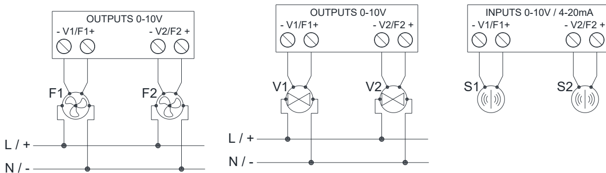
Abbildung 2: Verdrahtungsbeispiele
