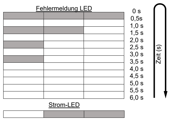
Abbildung 2: Fehlermeldungscode mit LEDs
