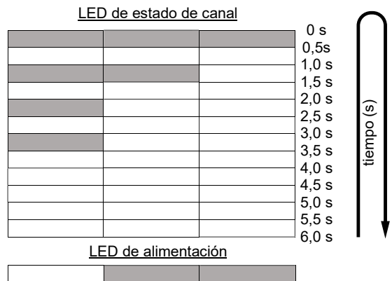
Figura 2: Códigos de notificación de error con LED
