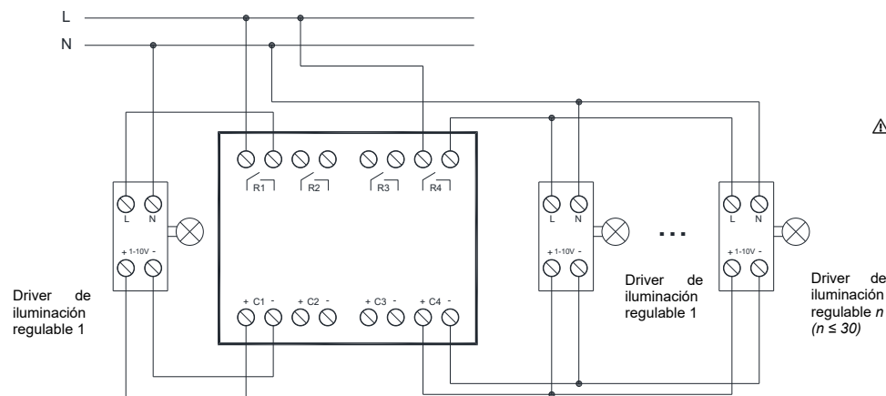
Figura 2: (de izquierda a derecha) Ejemplos de conexionado para un driver y varios drivers en paralelo
