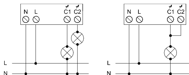
Figura 2: Ejemplos de conexionado (conexión de canales individuales y de canal común)
