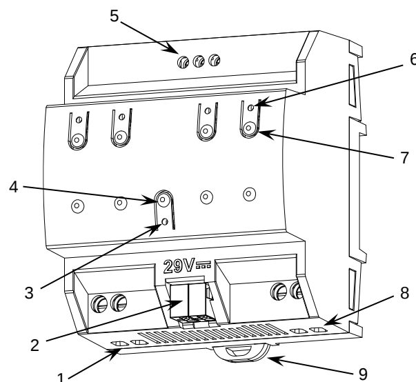
Figura 1: DIMinBOX DX2
