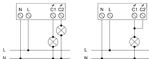
Figure 2 : Exemples de connexion (connexion des canaux individuels et d'un canal commun)
