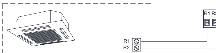
Figure 2 : Câblage du KLIC-PA à l'appareil de climatisation
