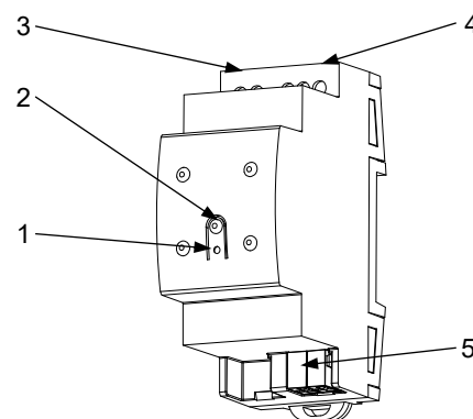
Figura 1: KLIC-DI v2
