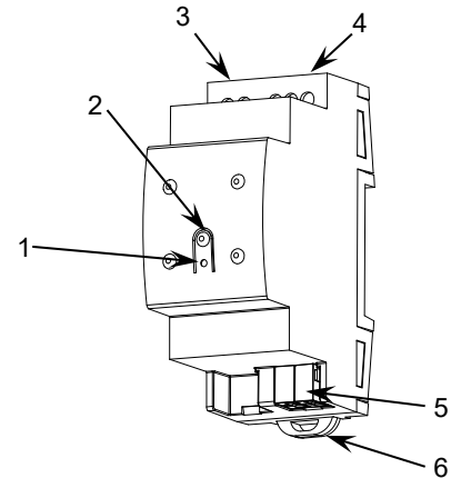
Abbildung 1: KLIC-DA v2
