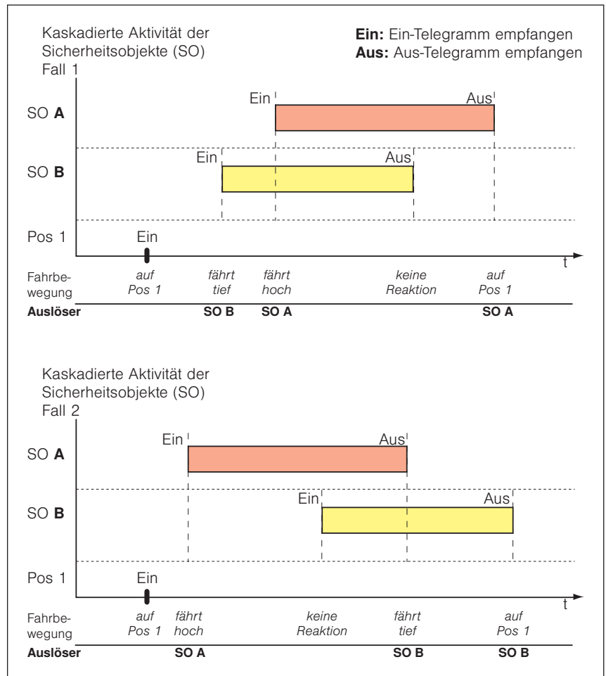
Abb. 54 Beispiel: Verhalten der Sicherheitsobjekte
