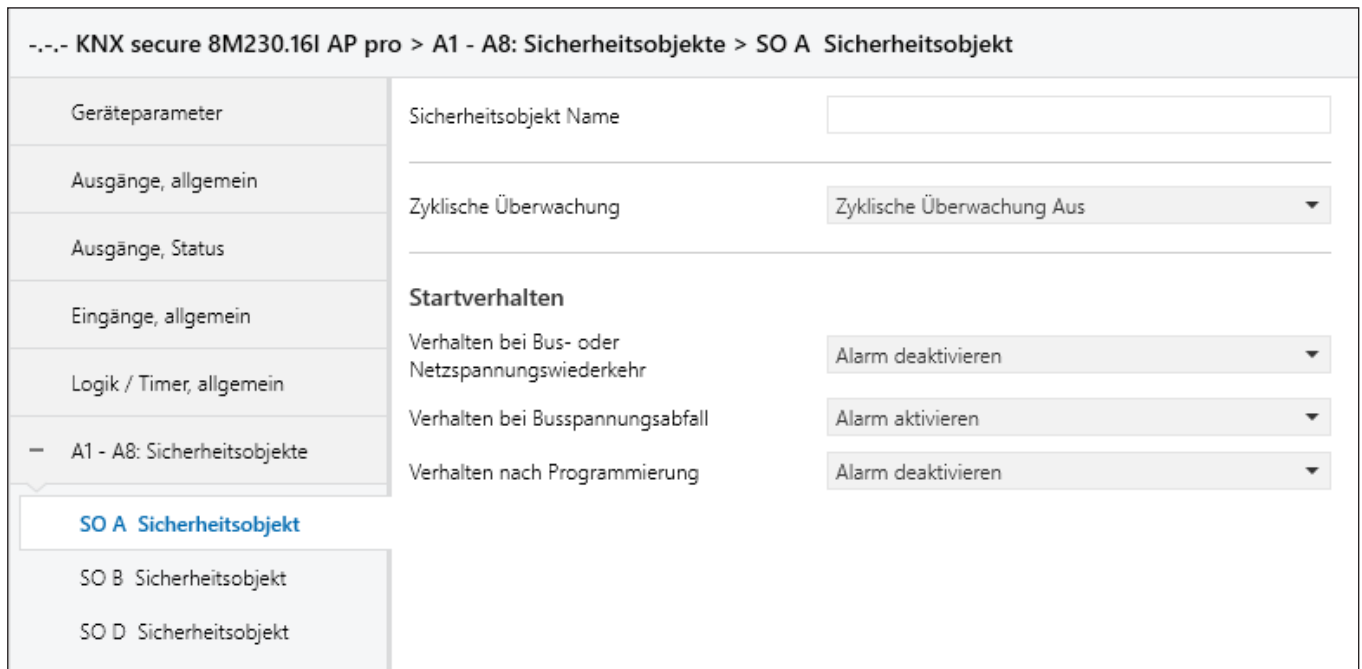
Abb. 55 Parameterdialog: Sicherheitsobjekte
