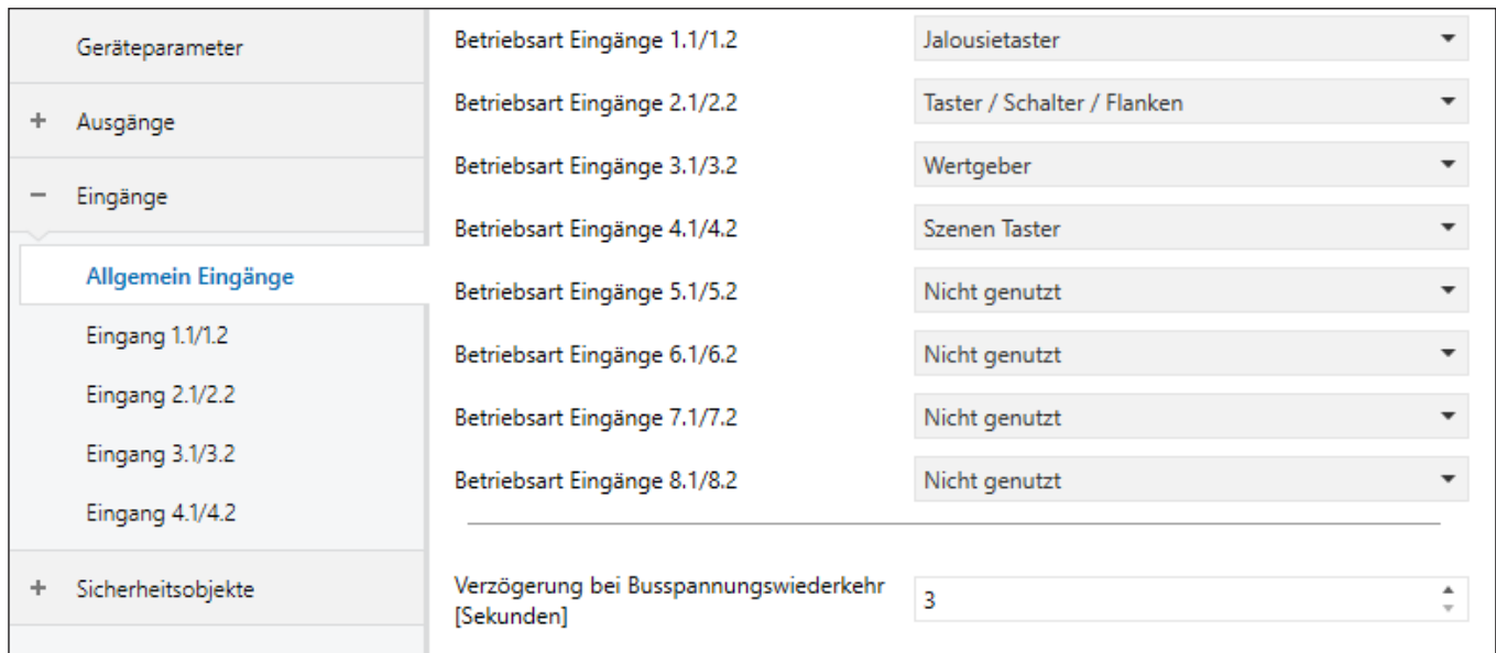
Abb. 28 Parameterdialog: Eingänge → Allgemein Eingänge
