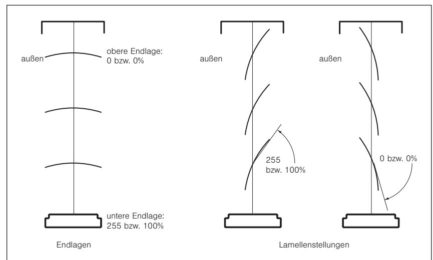
Abb. 7 Endlagen, Lamellenstellungen
