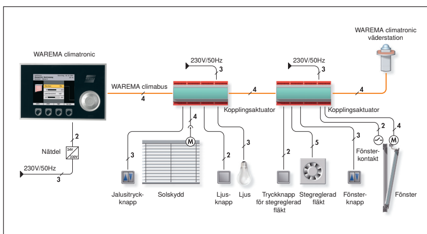
bild 1 Överblick över uppbyggnaden av ett WAREMA climatronic®-system
