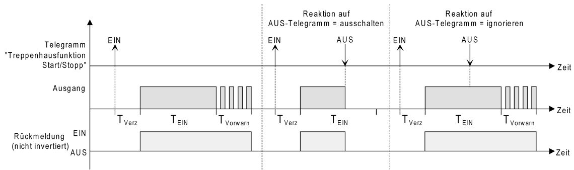
Bild 26: Ausschaltverhalten der Treppenhausfunktion
