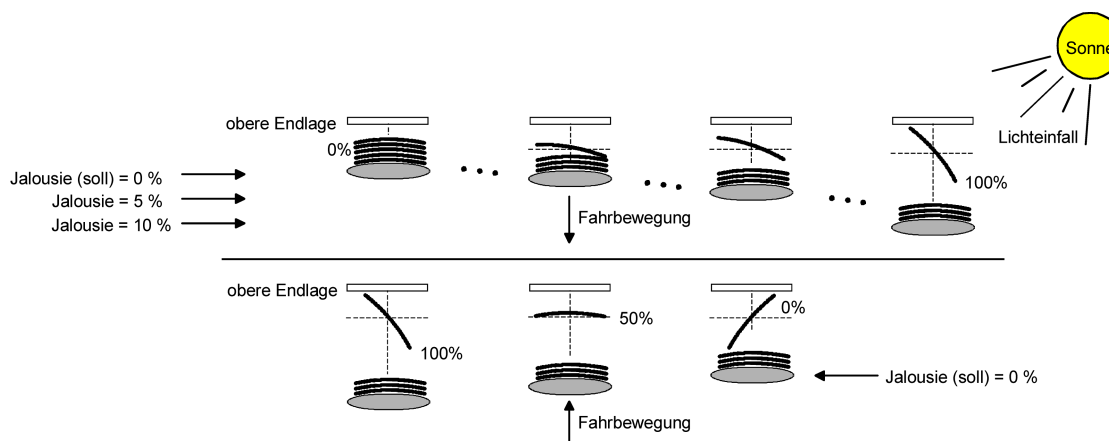
Bild 11: Beispiel für Lamellenpositionierung bei Jalousieposition in der oberen Endlage (Beispielhaft für Lamellentyp 1.)
