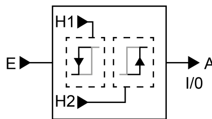
Bild 34: Grenzwertschalter
