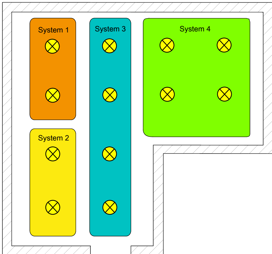
Bild 4: Beispiel einer Anordnung der DALI System im Großraumbüro
