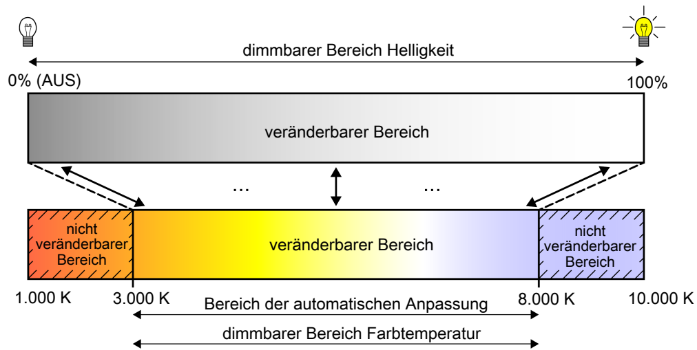
Bild 18: Automatische Anpassung der Farbtemperatur an die eingestellte Helligkeit Beispiel mit eingeschränktem Farbtemperaturbereich
