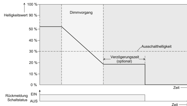
Bild 33: Dimm- und Schaltverhalten der automatischen Ausschaltfunktion
