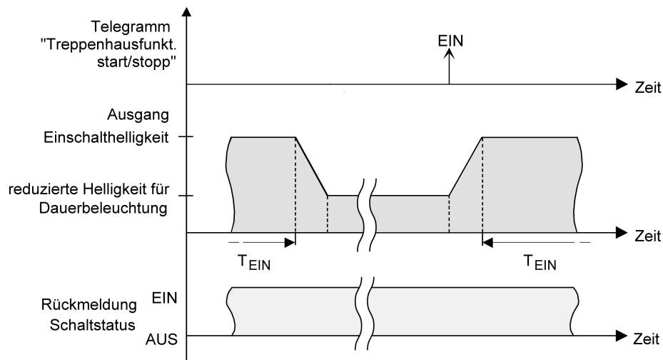
Bild 41: Die Dauerbeleuchtung der Treppenhausfunktion mit Soft-AUS-Funktion
