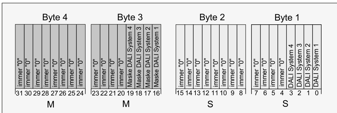
Bild 6: Struktur der Objekte der Sammelrückmeldung für die DALI Systeme 1-4
