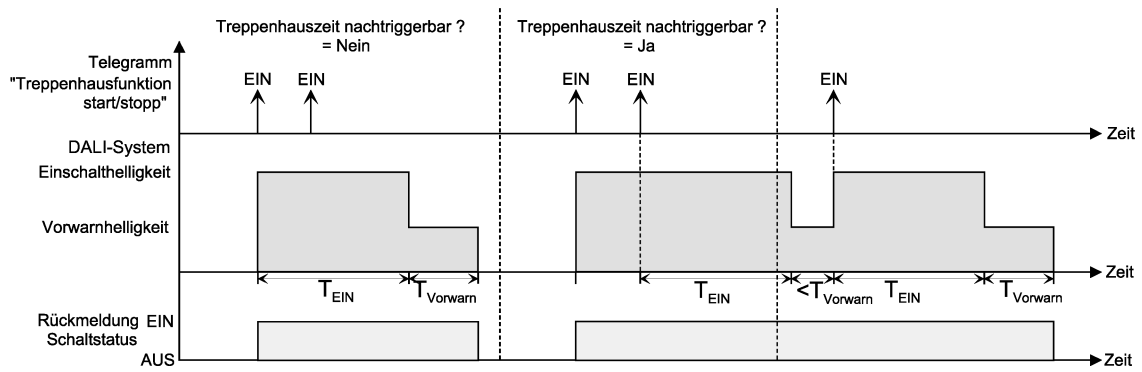
Bild 34: Einschaltverhalten der Treppenhausfunktion ohne Soft-Funktionen
