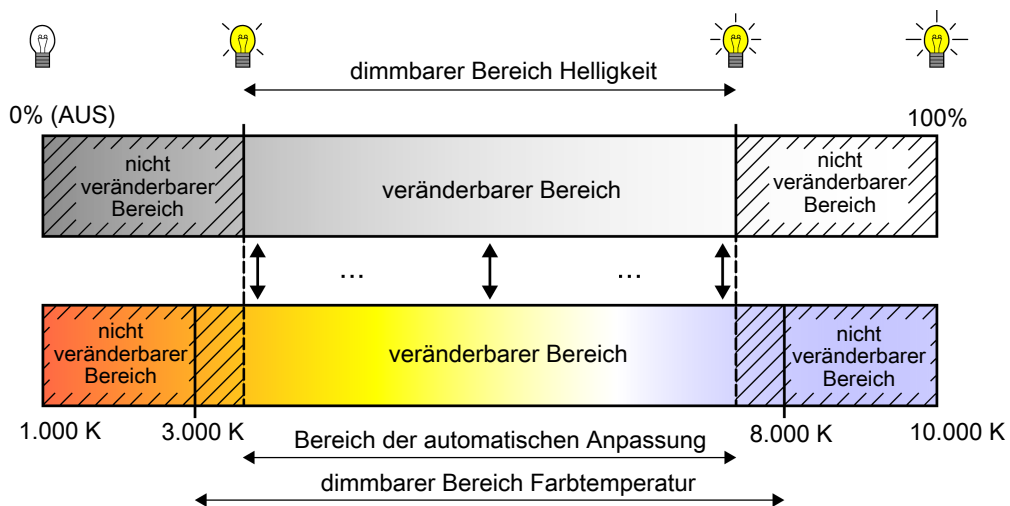
Bild 17: Automatische Anpassung der Farbtemperatur an die eingestellte Helligkeit Beispiel mit eingeschränktem Helligkeits- und Farbtemperaturbereich
