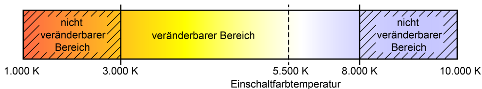
Bild 14: Beispiel eines konfigurierten Farbtemperaturbereichs mit Einschaltfarbtemperatur
