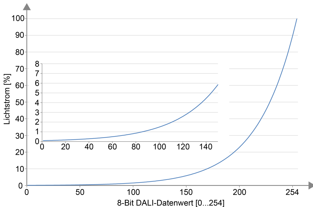
Bild 10: Logarithmische Dimmkurve in DALI Betriebsgeräten (relativer Lichtstrom [%] abhängig vom 8-Bit-DALI Datenwert [0...254])
