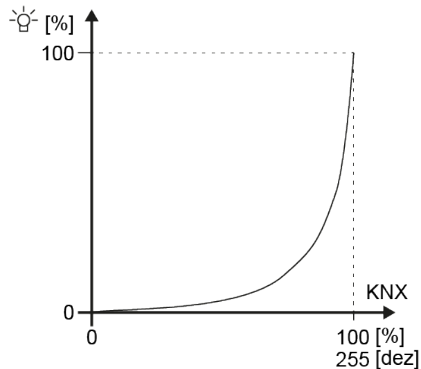
Bild 12: Logarithmische Dimmkennlinie am Ausgang eines Betriebsgeräts (relativer Lichtstrom [%] abhängig vom 8-Bit-KNX Datenwert [0...255])
