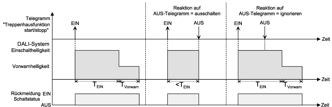
Bild 36: Ausschaltverhalten der Treppenhausfunktion ohne Soft-Funktionen
