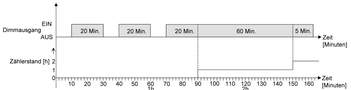
Bild 43: Funktionsweise des Betriebsstundenzählers (am Beispiel gezählter Stunden)
