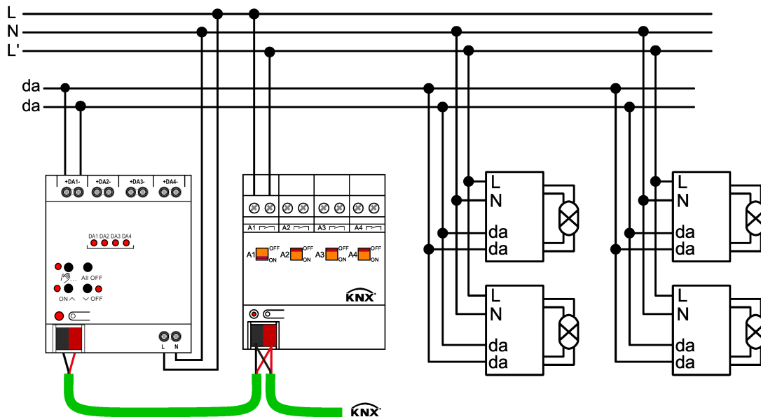
Bild 7: Beispiel eines Anschluss-Schemas zur Standby-Abschaltung durch einen KNX Schaltaktor
