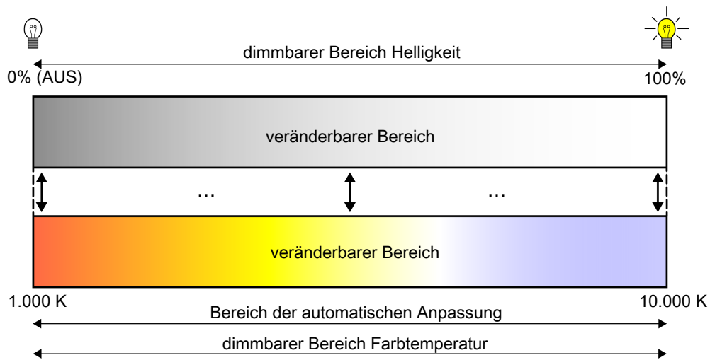
Bild 16: Automatische Anpassung der Farbtemperatur an die eingestellte Helligkeit Beispiel im maximalen Helligkeits- und Farbtemperaturbereich
