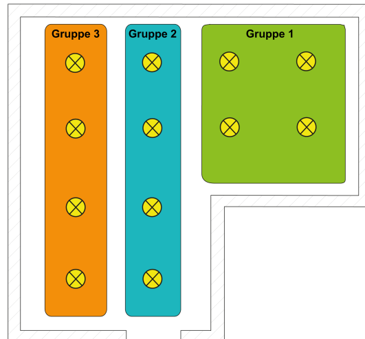
Bild 4: Beispiel einer Gruppensteuerung mit drei Gruppen - Alle Leuchten gruppen-adressiert
