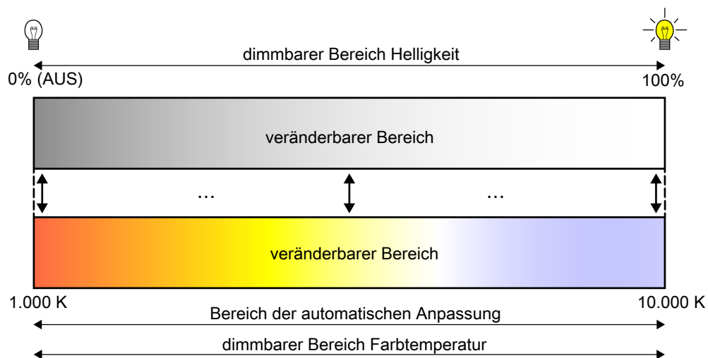
Bild 25: Automatische Anpassung der Farbtemperatur an die eingestellte Helligkeit Beispiel im maximalen Helligkeits- und Farbtemperaturbereich
