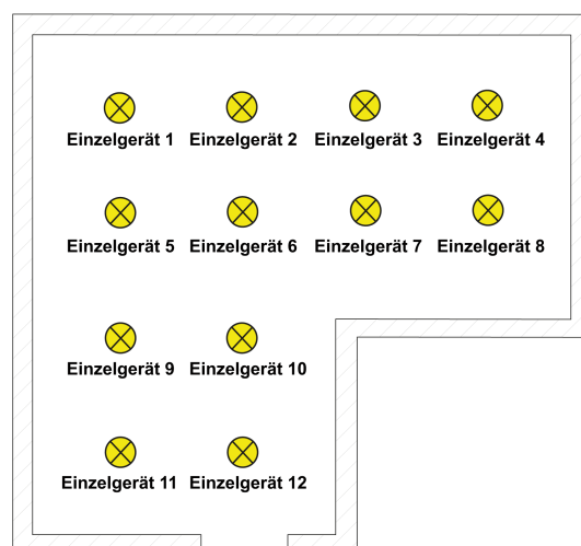
Bild 7: Beispiel einer Einzelgerätsteuerung - Alle DALI Betriebsgeräte individuell ansteuerbar
