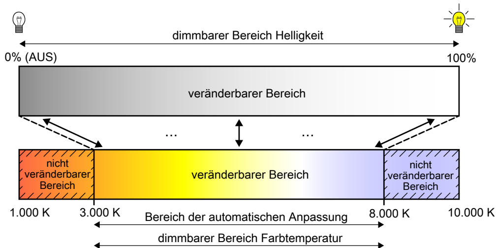
Bild 27: Automatische Anpassung der Farbtemperatur an die eingestellte Helligkeit Beispiel mit eingeschränktem Farbtemperaturbereich
