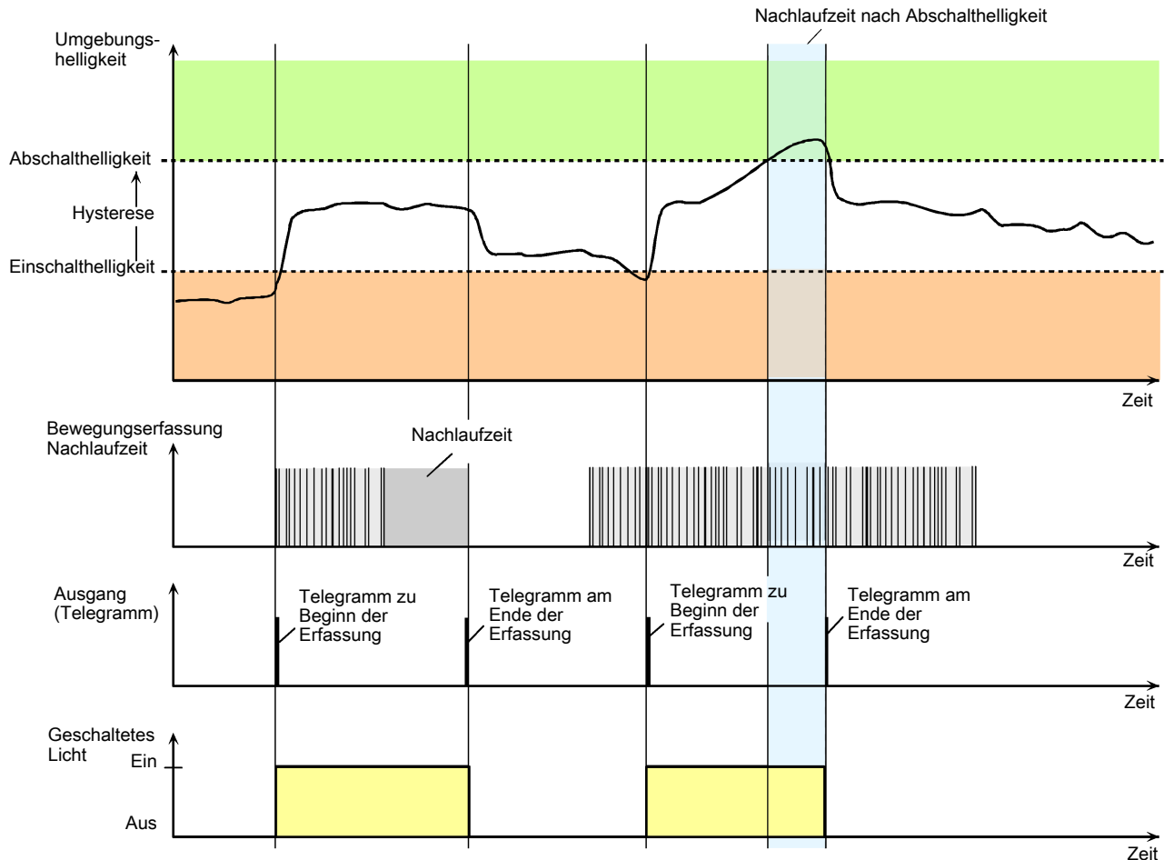
Bild 63: Helligkeitsabhängige Präsenzerkennung
