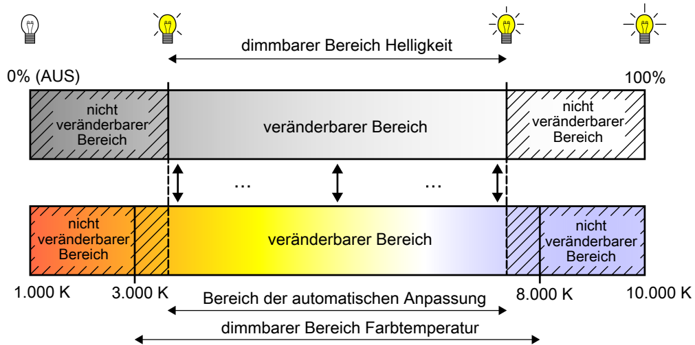
Bild 26: Automatische Anpassung der Farbtemperatur an die eingestellte Helligkeit Beispiel mit eingeschränktem Helligkeits- und Farbtemperaturbereich
