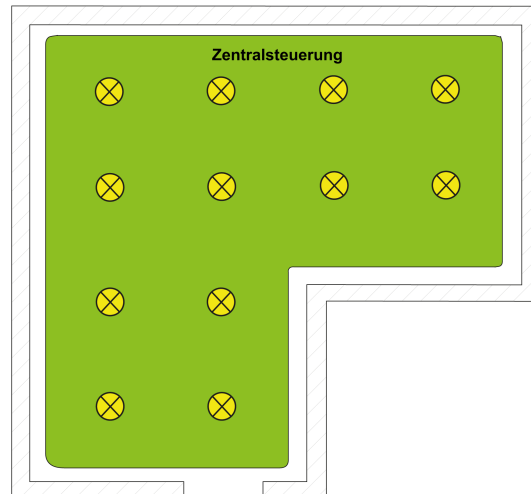
Bild 3: Beispiel einer Zentralsteuerung (Broadcast) - Nur eine Gruppe
