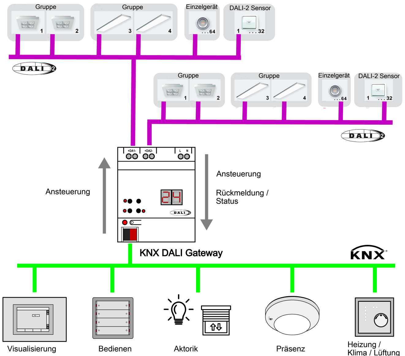
Bild 9: Prinzipübersicht einer KNX DALI Systemanbindung mit DALI Sensoren (Beispiel)
