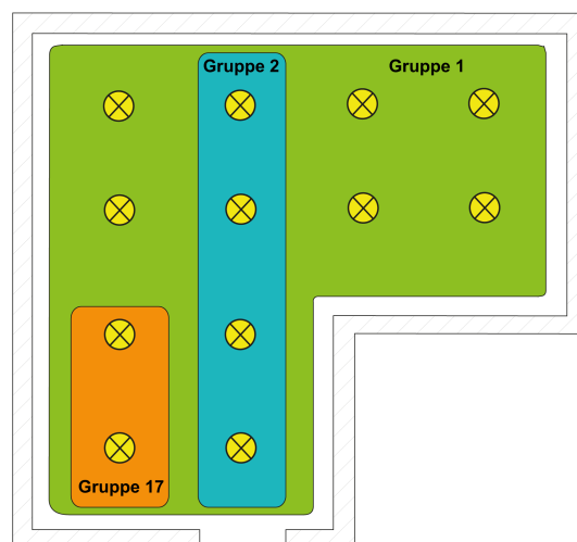
Bild 8: Beispiel einer Mehrfachzuordnung von Betriebsgeräten - Hier: Gruppe 1 überlappt Gruppe 2 und Gruppe 17
