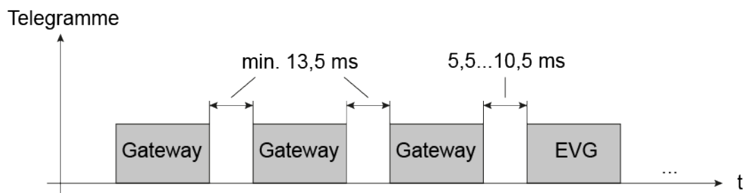
Bild 12: Pausenzeiten zwischen DALI Befehlen
