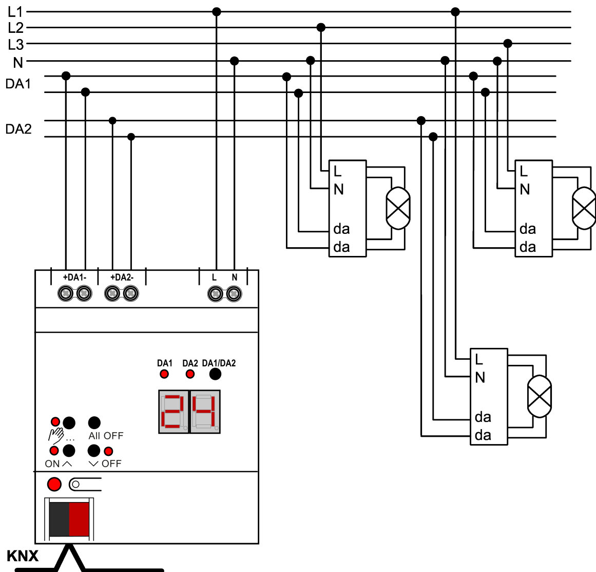
Bild 1: Anschlussbeispiel DALI Gateway 2fach
