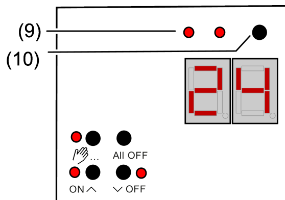
Bild 11: Bedienfeld DALI Gateway 2fach
