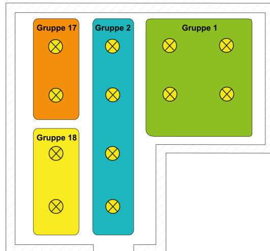
Bild 5: Beispiel einer Gruppensteuerung mit vier Gruppen - Leuchten in Gruppen 17 und 18 einzeln adressiert
