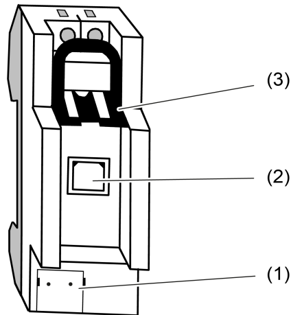
Bild 1: Geräteaufbau
