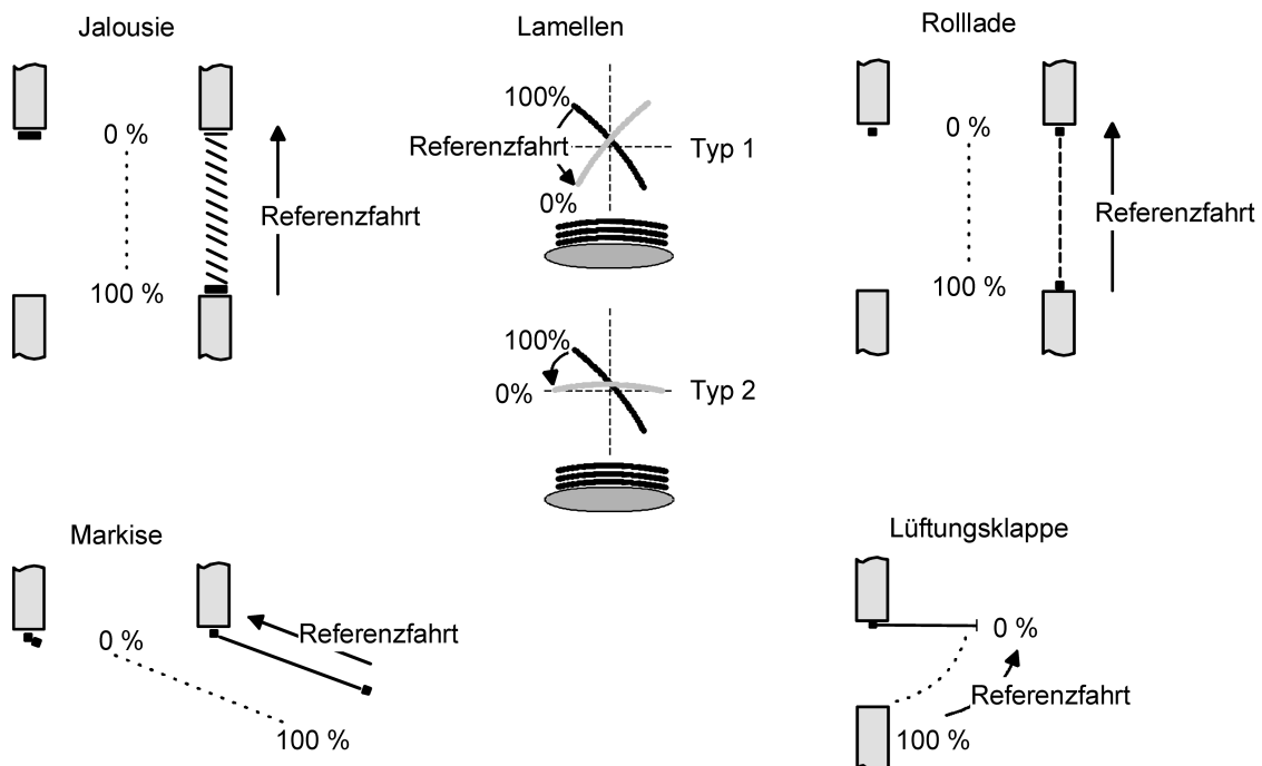
Bild 12: Referenzfahrt
